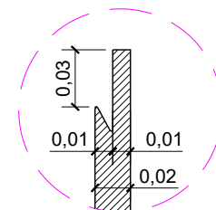
DET.02 - PUXADOR CAVA SEM ESCALA
