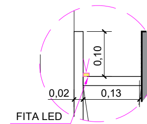
DET.05 - CORTINEIRO ILUMINADO
