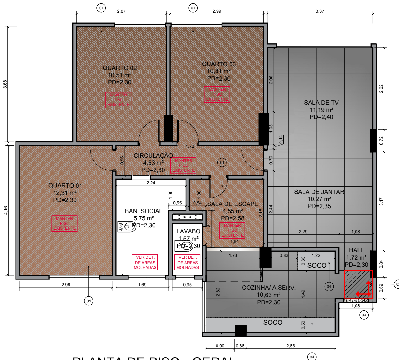
PLANTA DE PISO - GERAL 1:75
