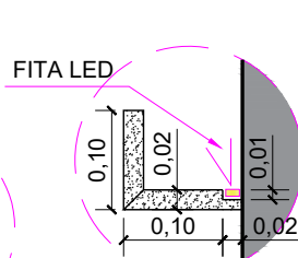
DET.03 - PORTA SHAMPOO LINEAR SEM ESCALA
