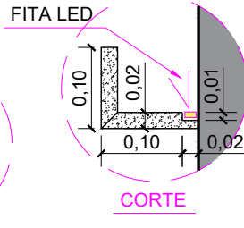
DET.03 - PORTA SHAMPOO LINEAR SEM ESCALA
