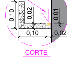
DET.03 - PORTA SHAMPOO LINEAR SEM ESCALA
