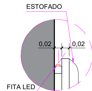
DET.01 - LED CABECEIRA
