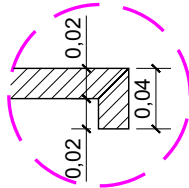
DET.01 - BANCADA SECA SEM ESCALA
