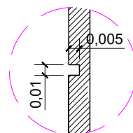
DET.06 - BITE
