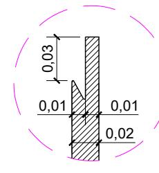
DET.04 - PUXADOR CAVA
