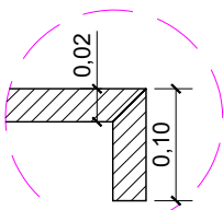
DET.01 - BANCADA SEM ESCALA
