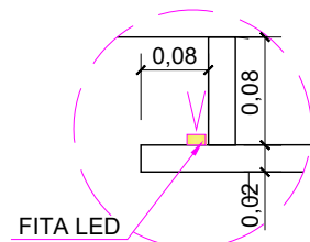
DET.02 - LED TETO PÓRTICO
