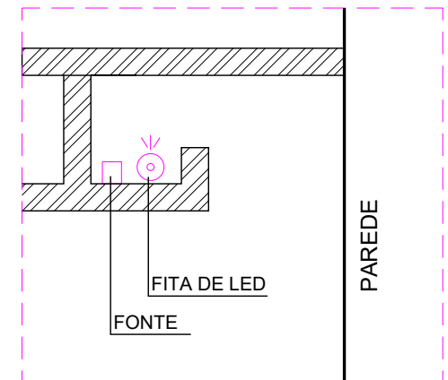
DET.01- FORRO/ CORTINEIRO ILUMINADO
