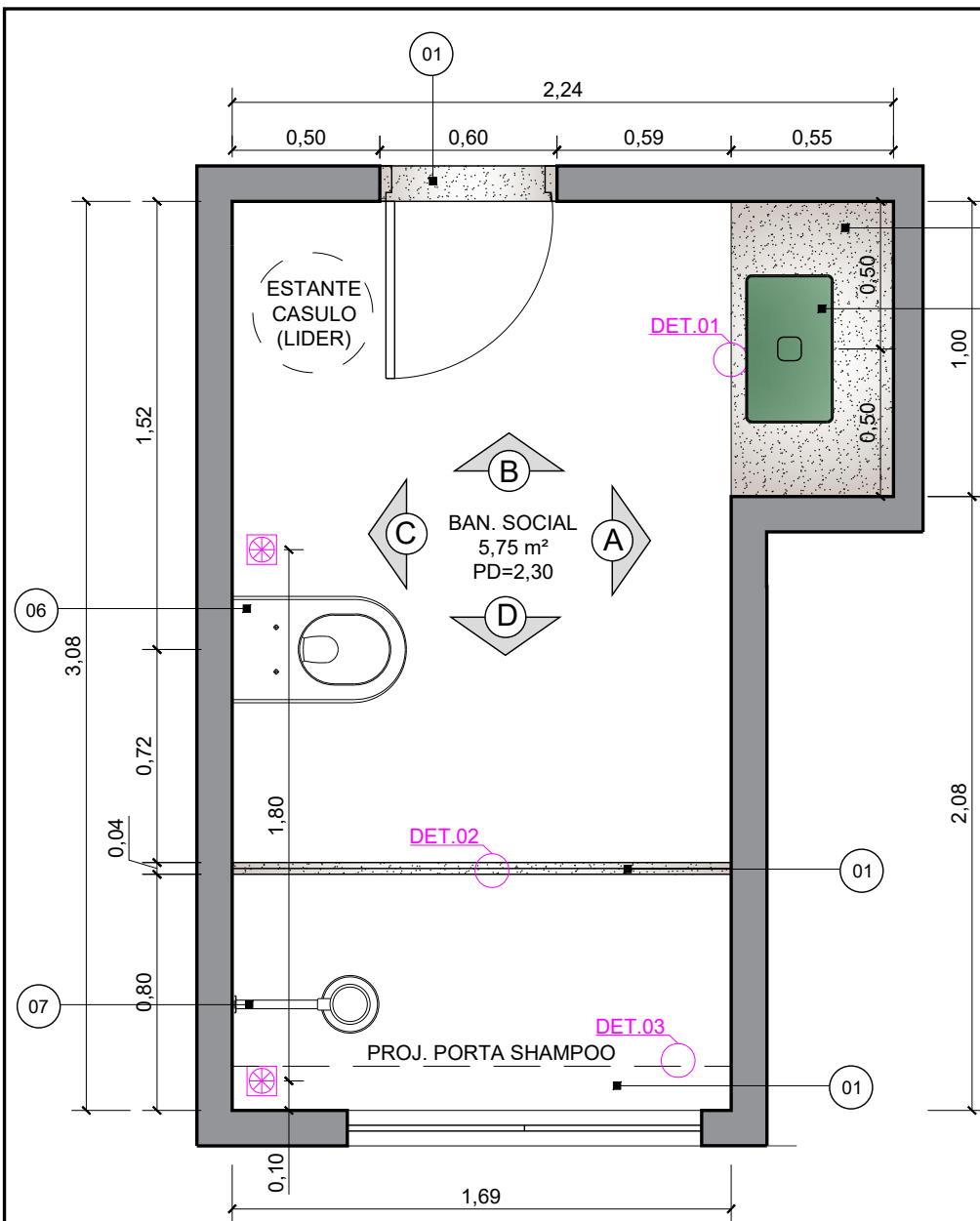
PLANTA BAIXA - BAN. SOCIAL
