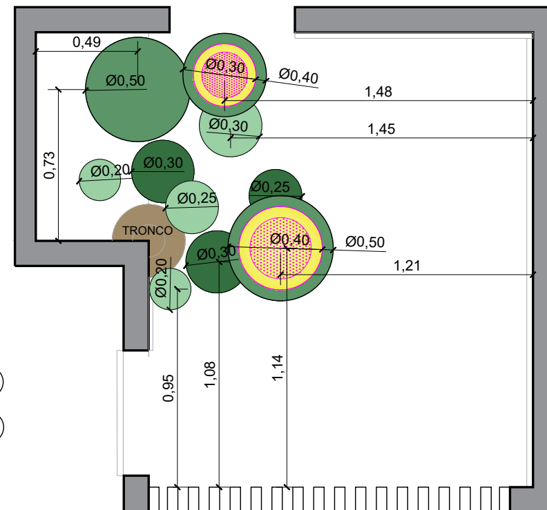
PLANTA TETO - FOLHAS ÁRVORE
