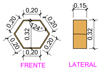
DETALHE - PRAT. EM ACM
