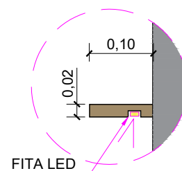
DET.04 - LED PRATELEIRA SEM ESCALA
