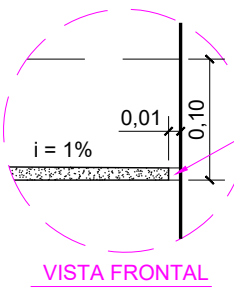
DET.03 - PORTA SHAMPOO LINEAR SEM ESCALA
