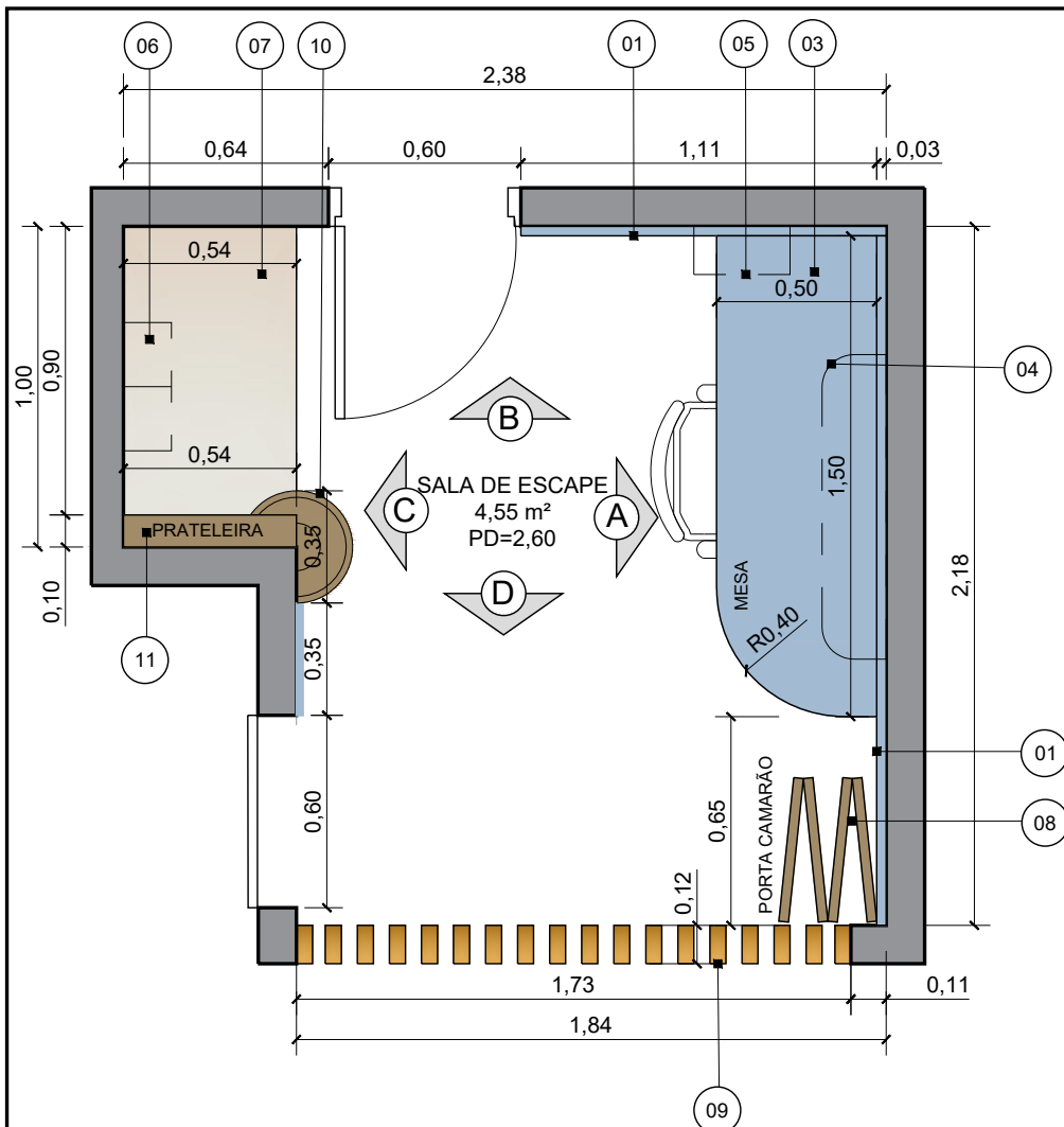
PLANTA BAIXA - SALA DE ESCAPE
