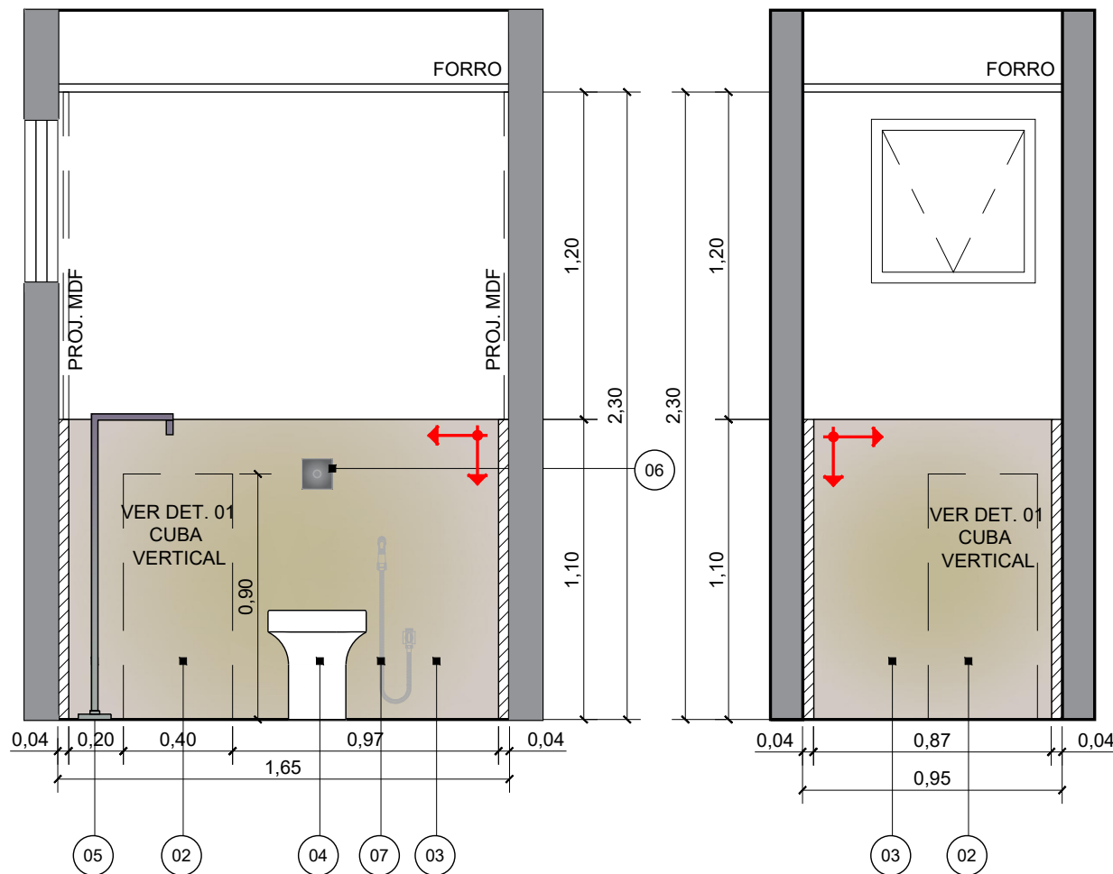
VISTA A - LAVABO
