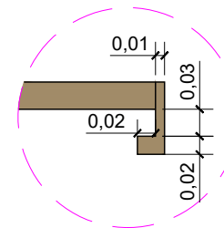
DET.05 - PUXADOR L SEM ESCALA
