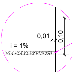
DET.03 - PORTA SHAMPOO LINEAR SEM ESCALA
