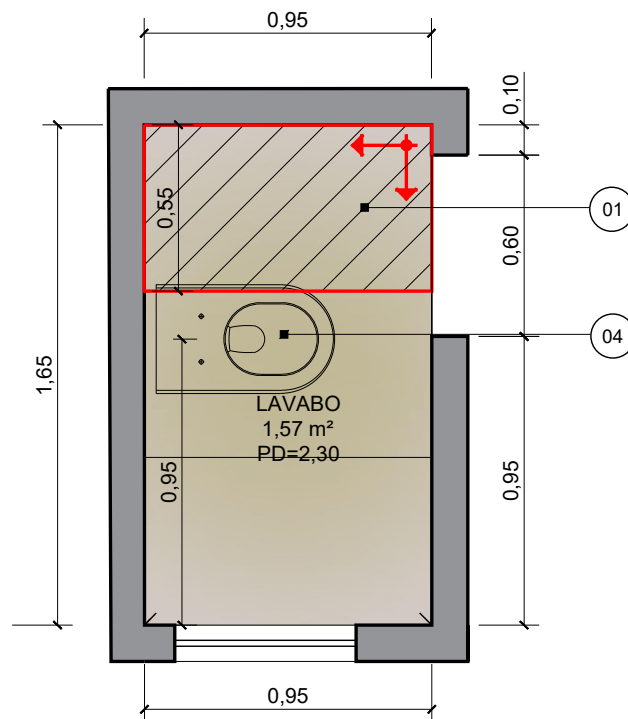
PLANTA DE PISO - LAVABO
