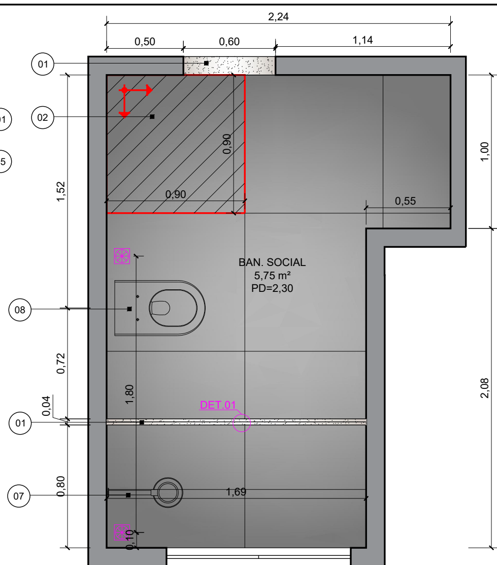
PLANTA DE PISO - BAN. SOCIAL
