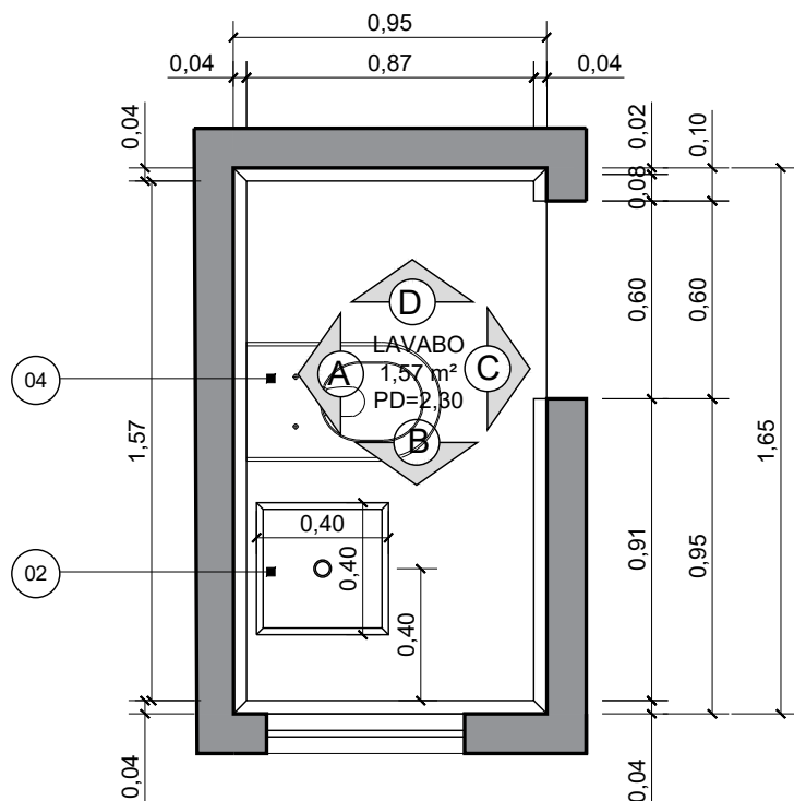
PLANTA BAIXA - LAVABO
