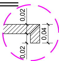
DET.01 - BANCADA SECA SEM ESCALA
