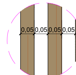
DET.06 - ESPAÇAMENTO BRISE SEM ESCALA
