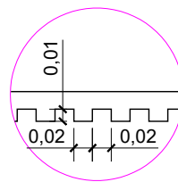
DET.03 - RIPADO
