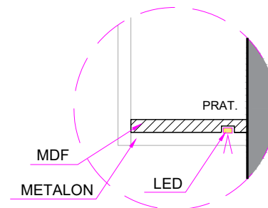
DET.01 - LED PRAT. METALON SEM ESCALA
