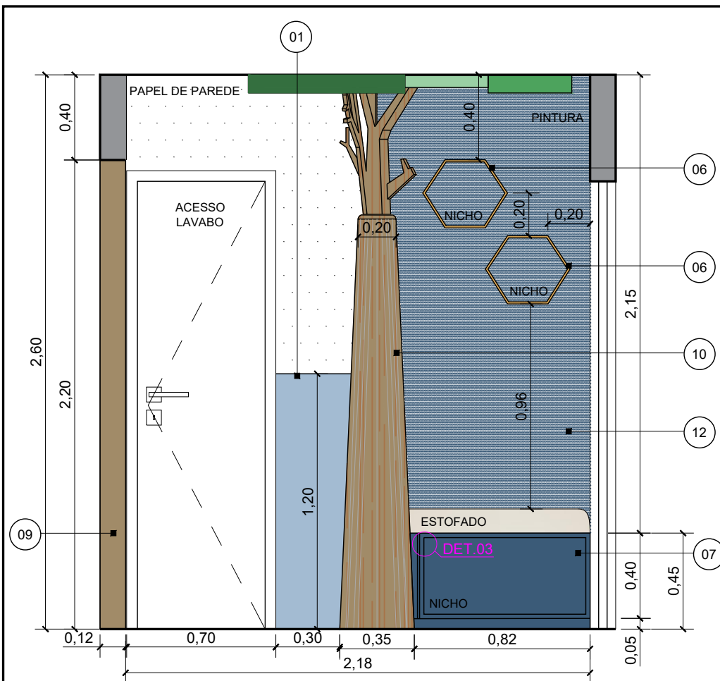
VISTA C - SALA DE ESCAPE
