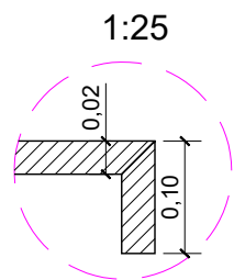
DET.01 - BANCADA SEM ESCALA
